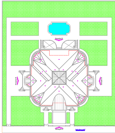
Implantação e Cobertura
